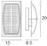
VL-5-C029/W E14 x 1
